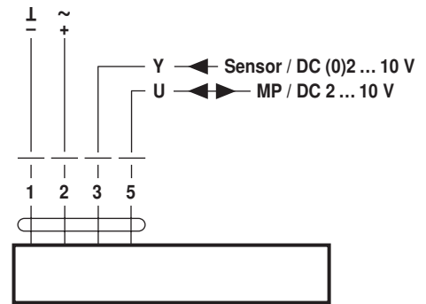
EF24A-MP / EF24G-MP
